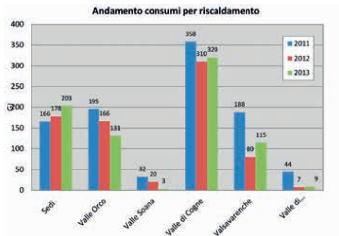
Grafico 5. Andamento consumi di carburante per riscaldamento e acqua calda sanitaria per il periodo 2011-2013
