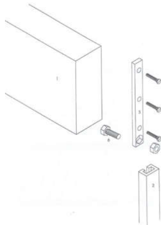
PARTICOLARE ANCORAGGIO CARTELLO
