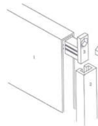
PARTICOLARE ANCORAGGIO CARTELLO
